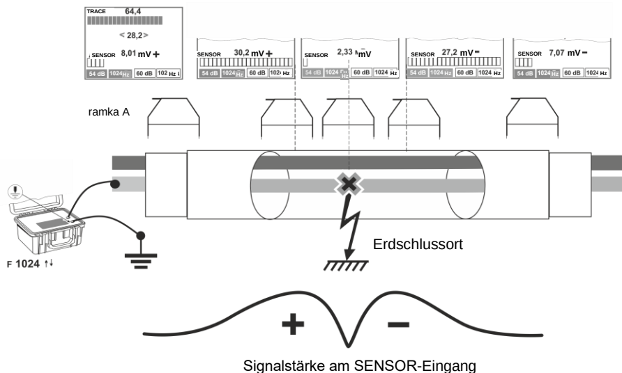
Abb. 38. Anschlusschema und Signalstärke für die Methode der Isolationsschadenverfolgung mit Isolationskontrolle
