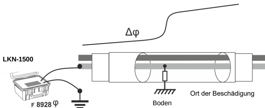
Abb. 39. Anschlusschema und Phasenverschiebung bei der Phasenmethode der Lokalisierung von Kabelisolierungsfehlern
