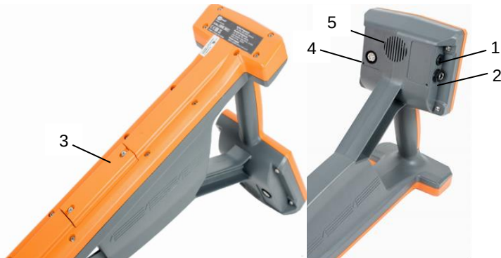
Abb. 7. Äußeres und Kennzeichnung der Empfängerbuchsen
