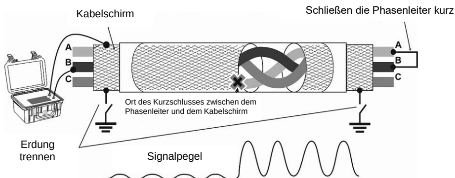
Abb. 37. Layout und Signalstärke der Verfolgung eines Leiter-Panzer-Kurzschlusses
