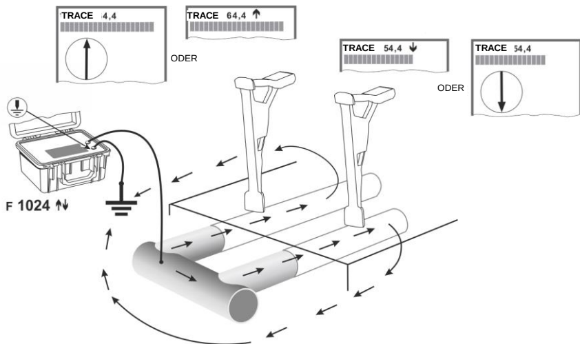
Abb. 27. Die Stromrichtung in den galvanisch gekoppelten benachbarten Leitungen
